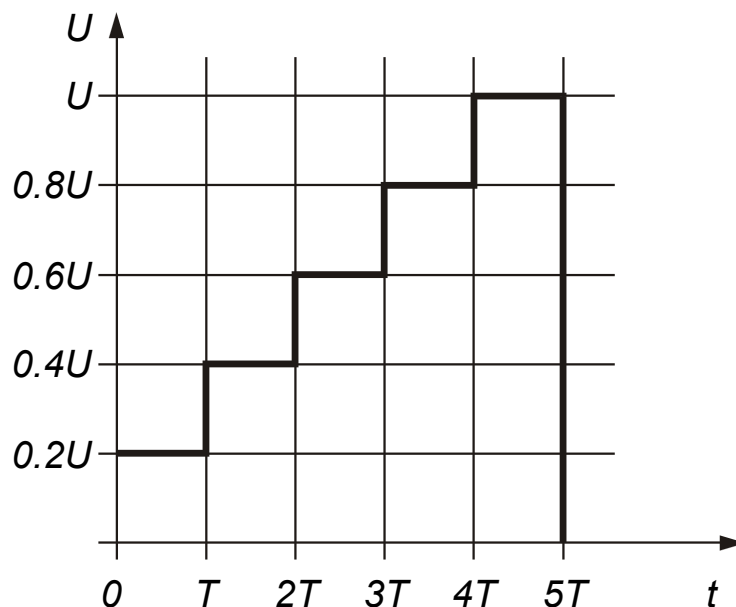
Fig. 23. Step-up test voltage
